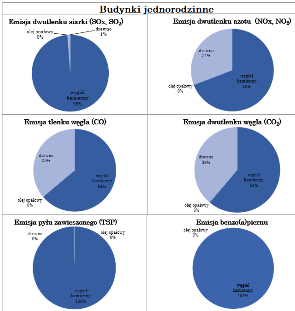
Rycina 14. Procentowy udział używanych źródeł ciepła w poszczególnej emisji zanieczyszczeń.
